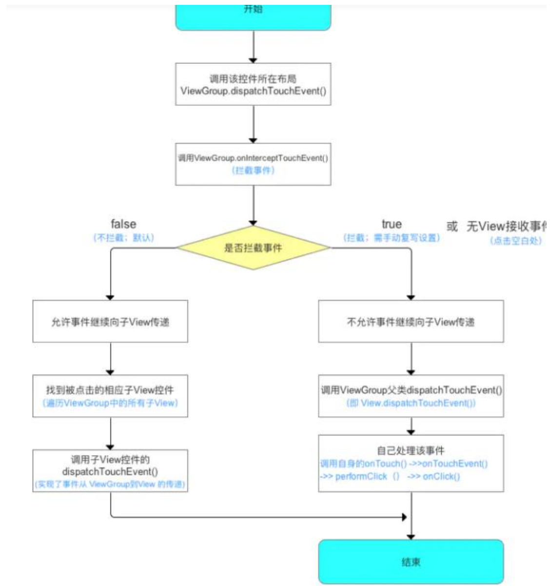
View 的事件分发示意图
