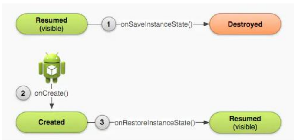
异常情况下activity的重建过程
